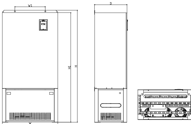
TVFE9-41850G TVFE9-46300G外形尺寸示意图
