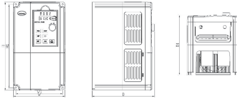
TVFE9-2007G TVFE9-2040G及TVFE9-4007G TVFE9-4110G外形尺寸示意图
