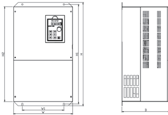
TVFE9-4150G TVFE9-41600G外形尺寸示意图
